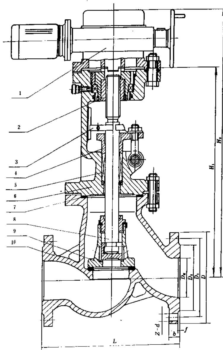
图 2-7 电动截止阀
