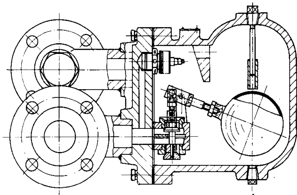
图 2-14 双阀座杠杆浮球式疏水阀
