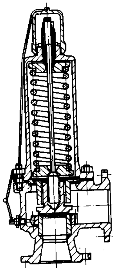
图 2-29 安全阀
