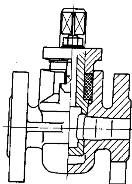
图 2-13 旋塞阀
