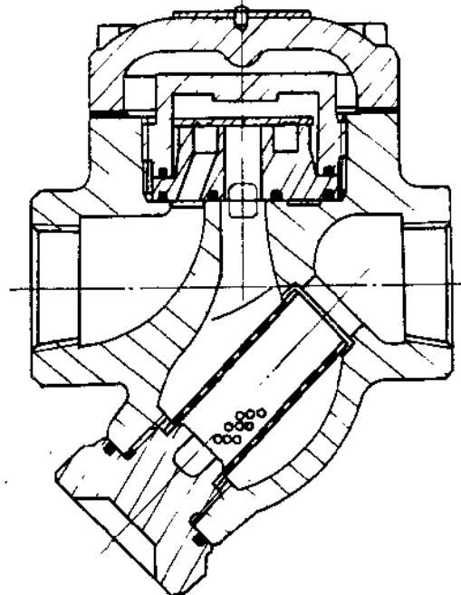
图 2-28 圆盘式疏水阀
