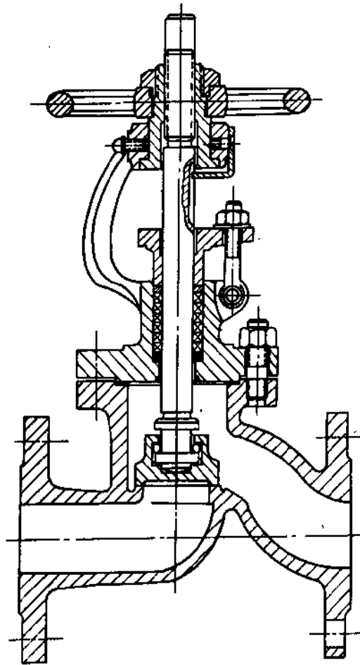
图 2-5 截止阀
