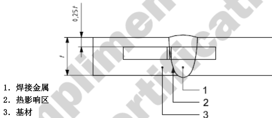
图 16—热影响区试样的夏比 V 形缺口摆锤试验位置
